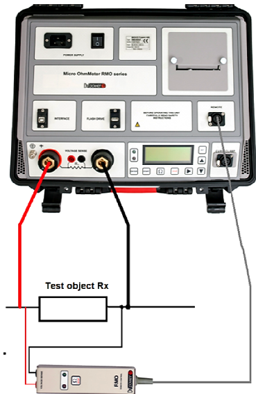
Рисунок 3 – Измерение с помощью блока дистанционного управления
