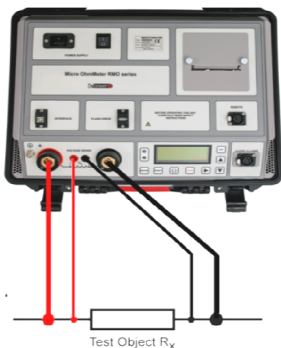
Рисунок 4 – Подключение к тестируемому объекту
