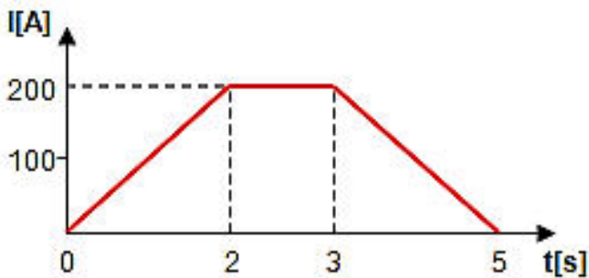
Рисунок 1 – Единичное линейное изменение
